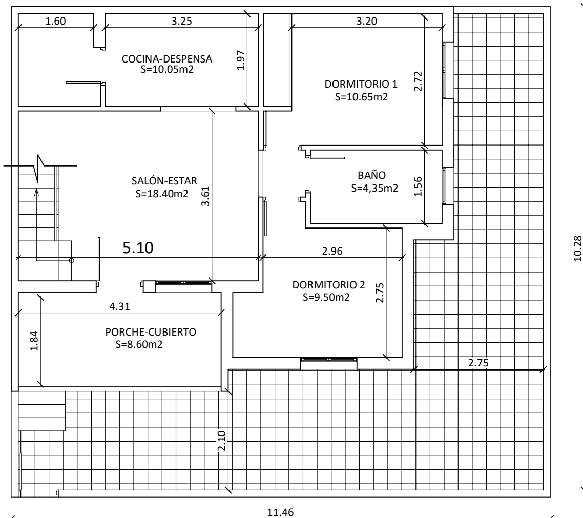
PLANTA BAJA SUP. CONSTRUIDA = 72.40 m 2
