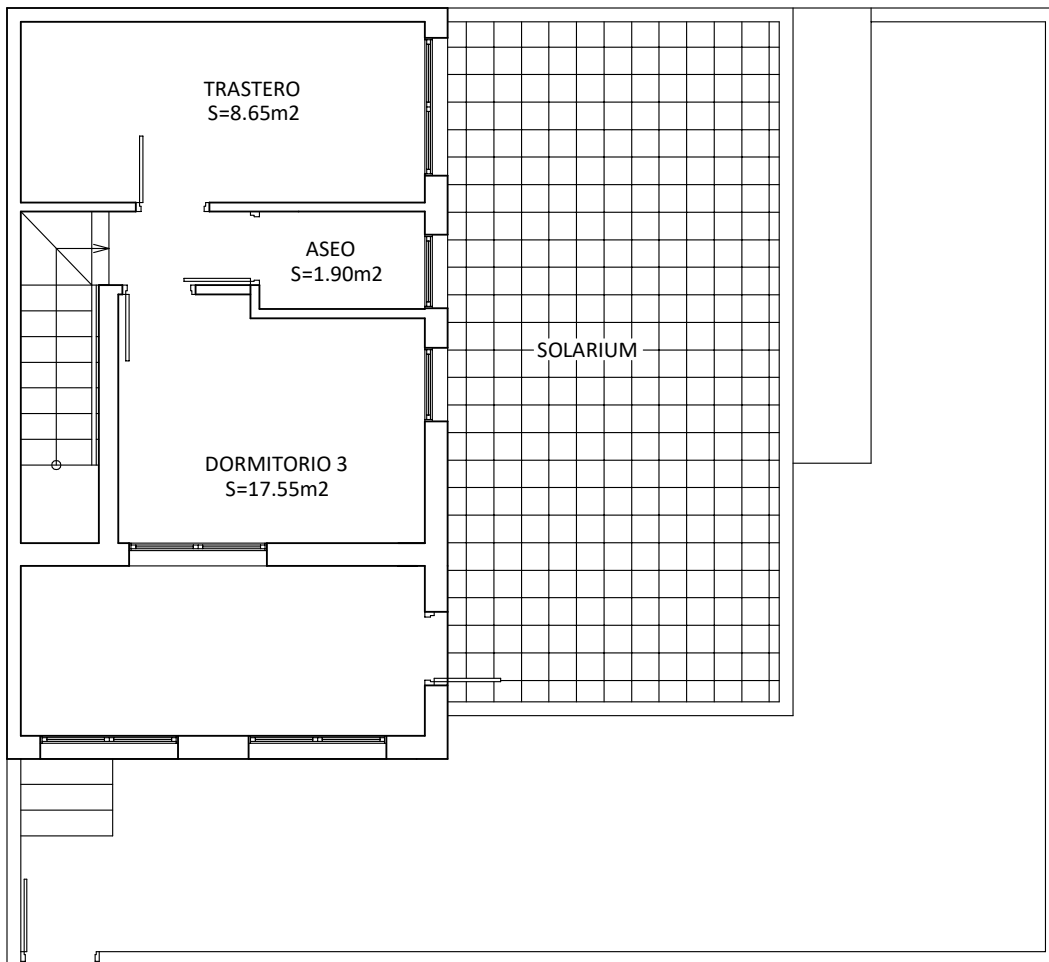
PLANTA ALTA SUP. CONSTRUIDA = 39.25 m 2
